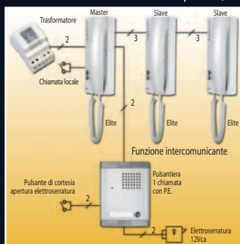
Kit unifamiliare - Installazione con citofoni in parallelo (slave)
