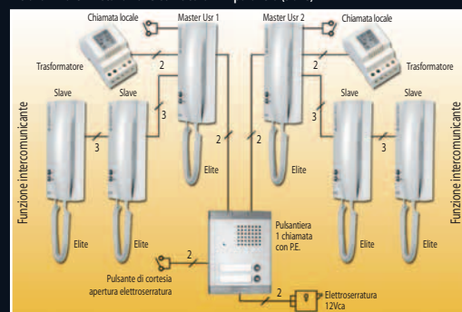
Kit bifamiliare - Installazione con citofoni in parallelo (slave)
